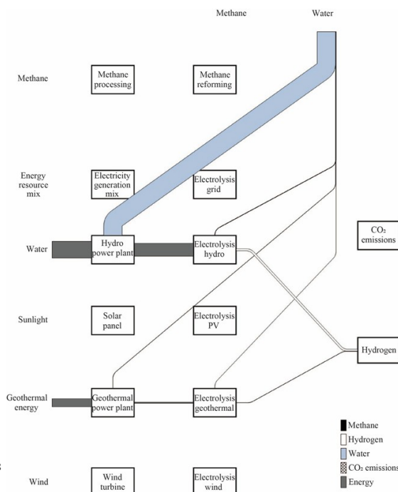
ベースシナリオにおける水素生成システムのエネルギーフローおよびマテリアルフロー (CO 2 強度 = 0 kg-CO 2 /kg-H 2 )
