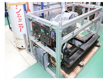
アンモニアによるエンジン発電
