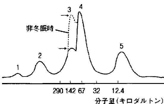
(図1) 冬眠中のシマリスから採取した血漿蛋白質を高速液体クロマトグラフィーによって分離した記録。破線は非冬眠時に採血した血漿の記録で、冬眠中には第3番目のピークが大きく低下していることがわかる。下線の数値は、蛋白質の分子量の目安(標準試料の分子量)。
